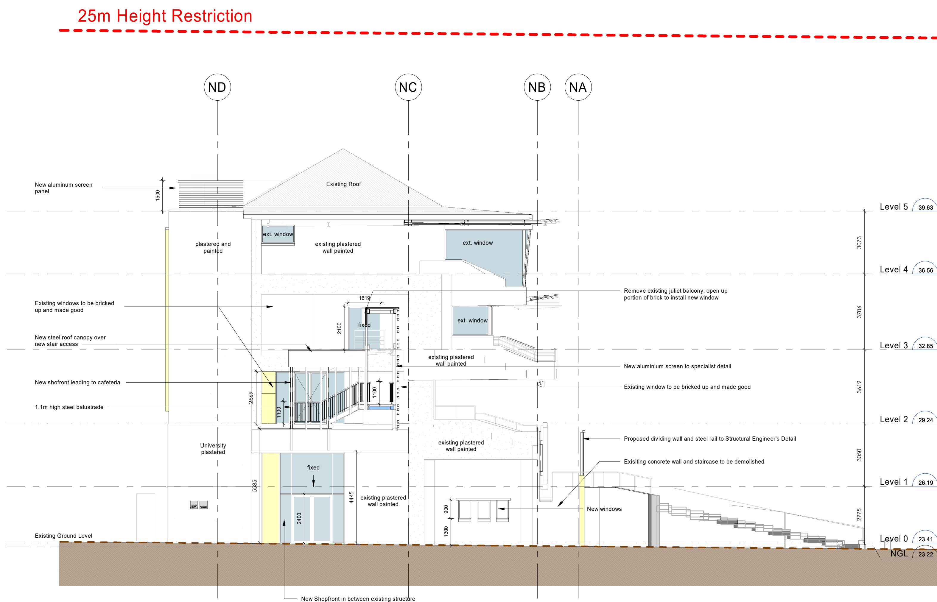
3 LA West Elevation SCALE: 1 : 100
