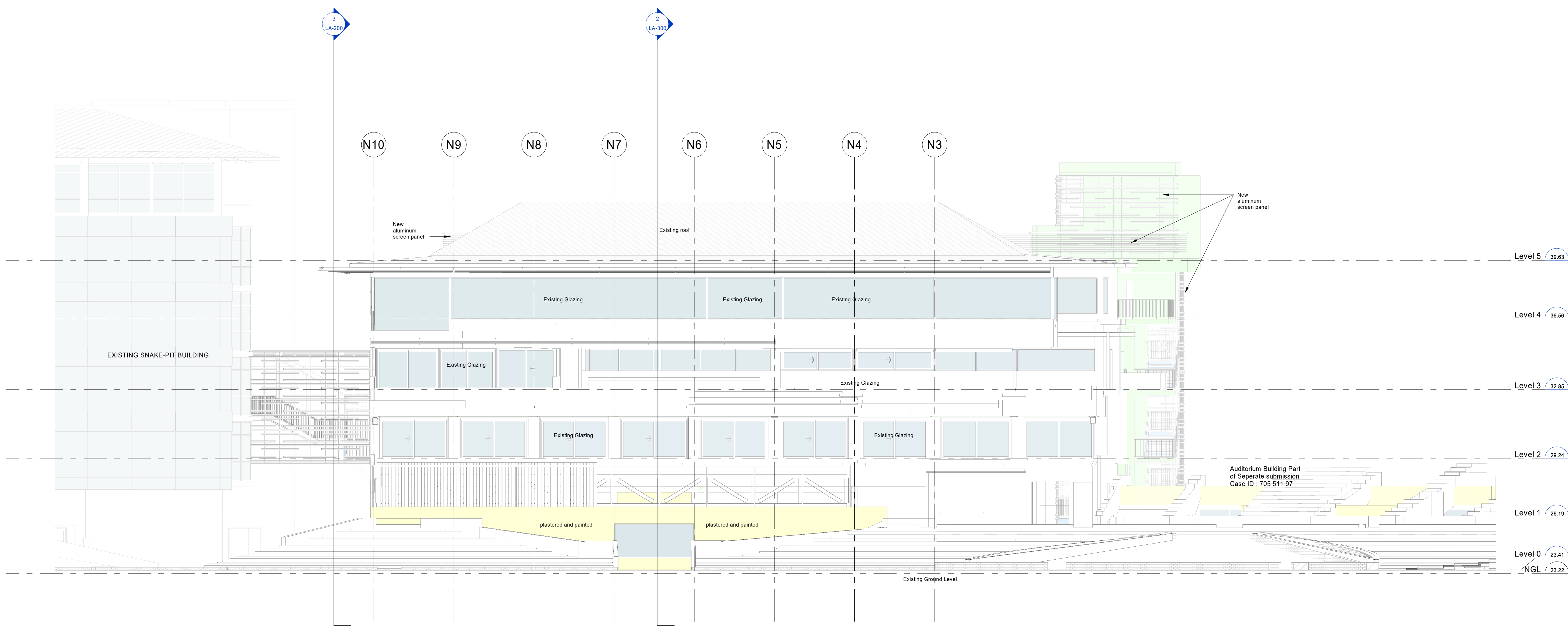
1 LA South Elevation SCALE: 1 : 100
