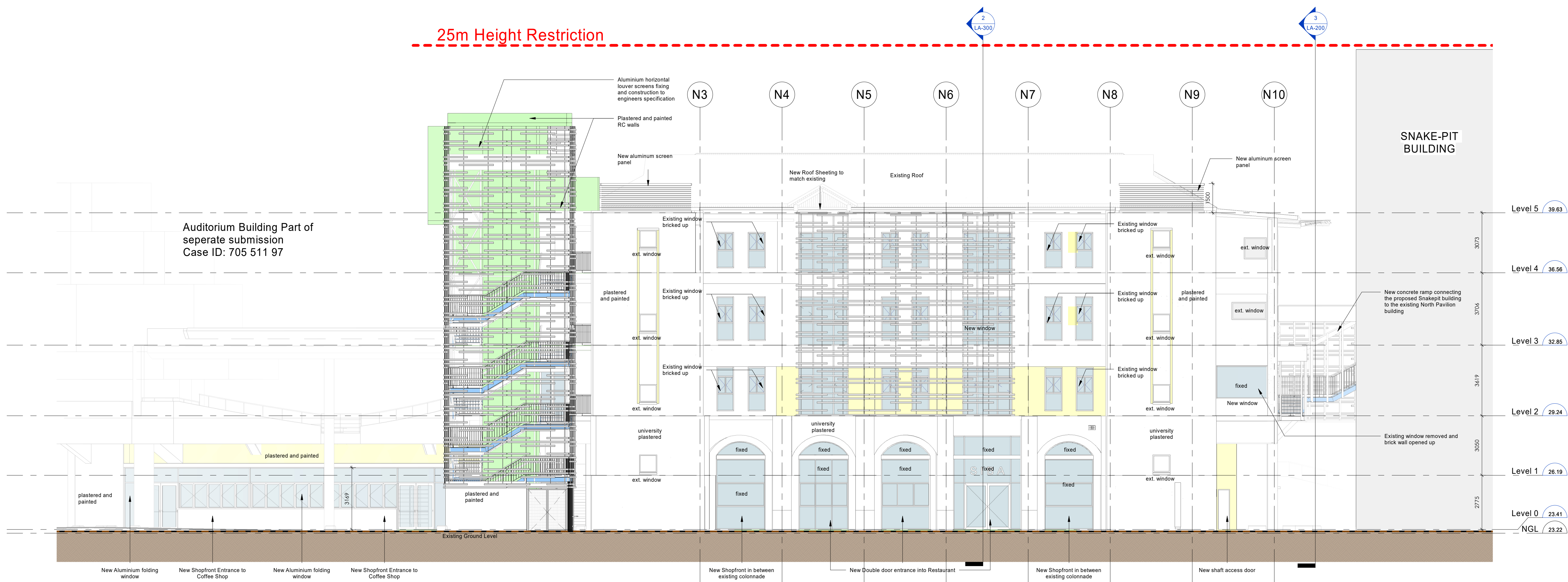
1 LA North Elevation SCALE: 1 : 100
