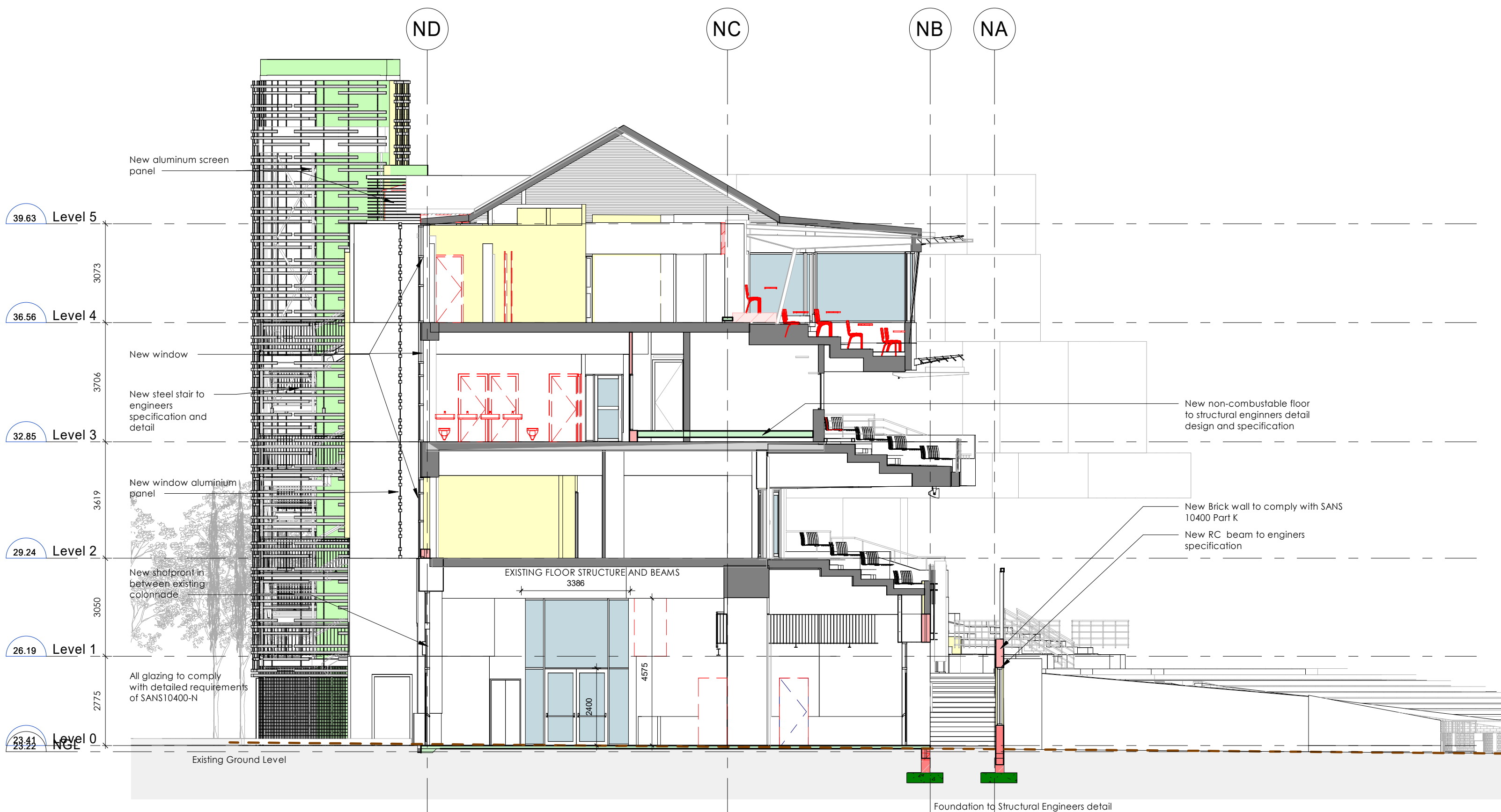
2 LA_SECTION B-B SCALE: 1 : 100
