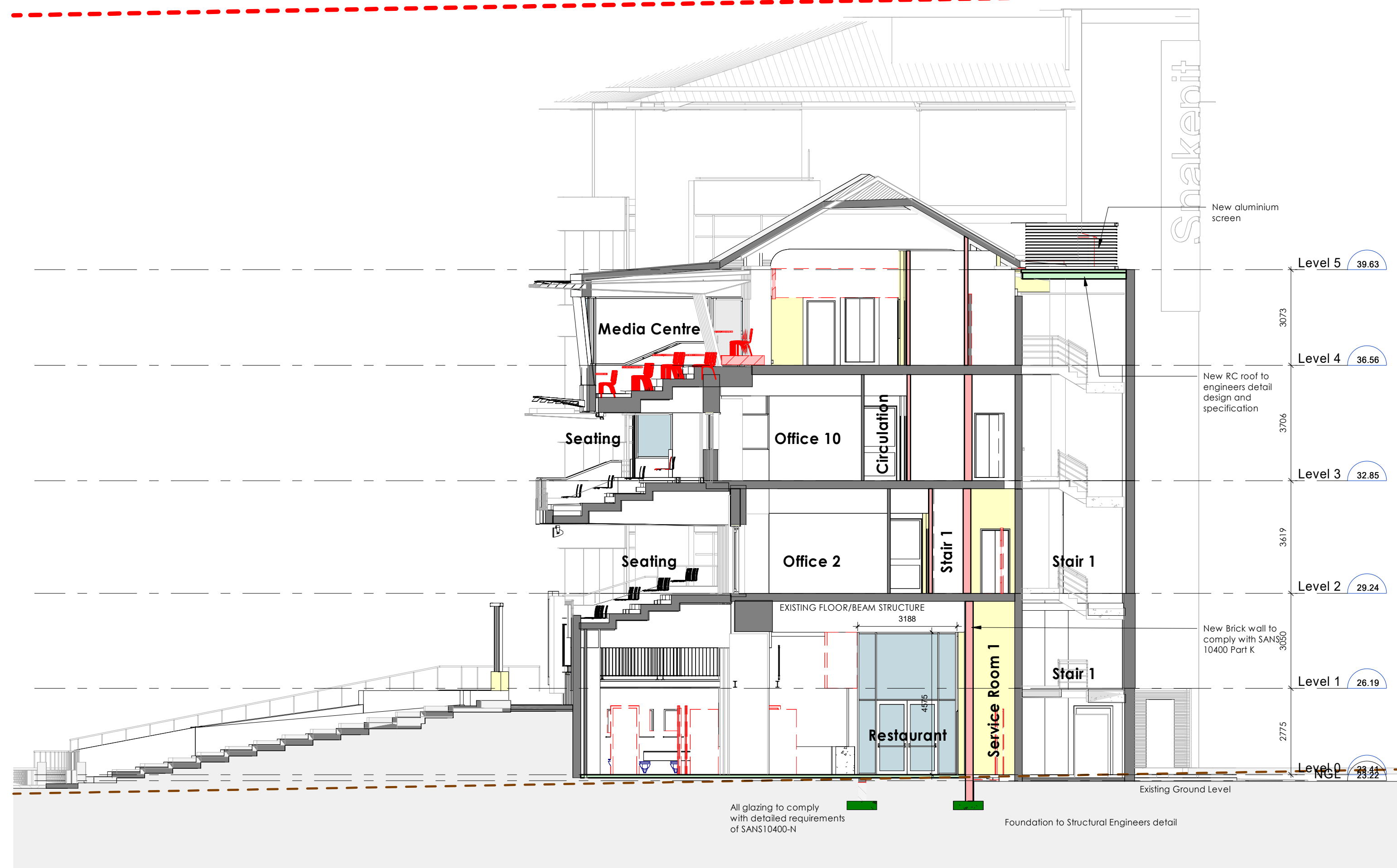
3 LA_SECTION C-C SCALE: 1 : 100
